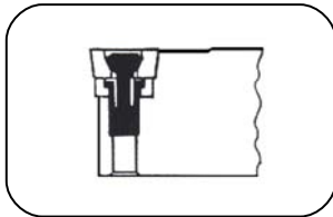
Fixation par vis Torx
